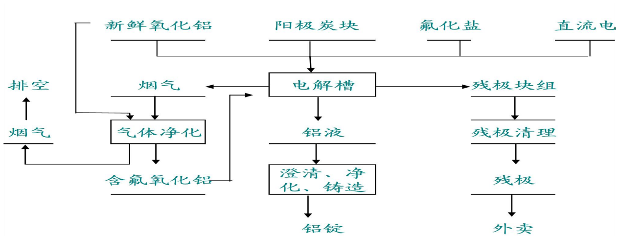
系统边界图
